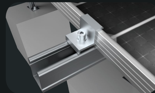
侧压块安装
