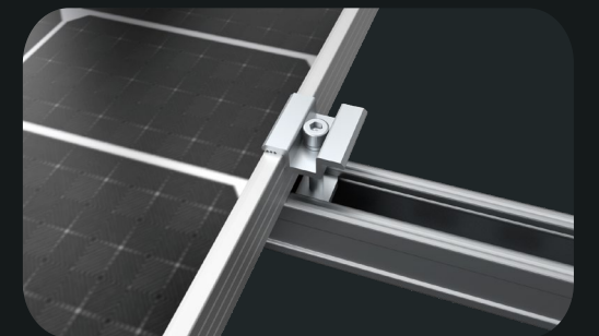
中压块安装
