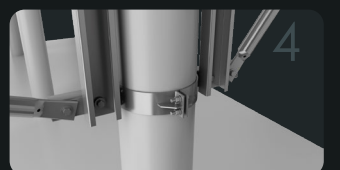
抱箍安装
