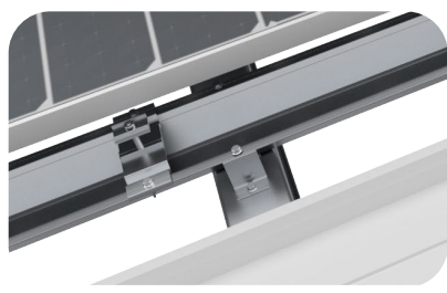
导水梁安装
