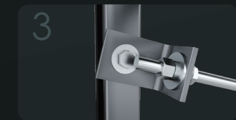
斜拉安装
