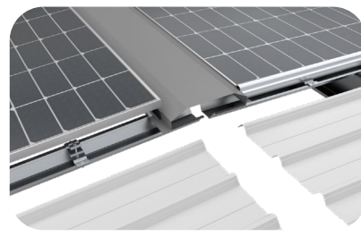
屋脊盖板安装
