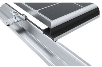
T型胶条安装
